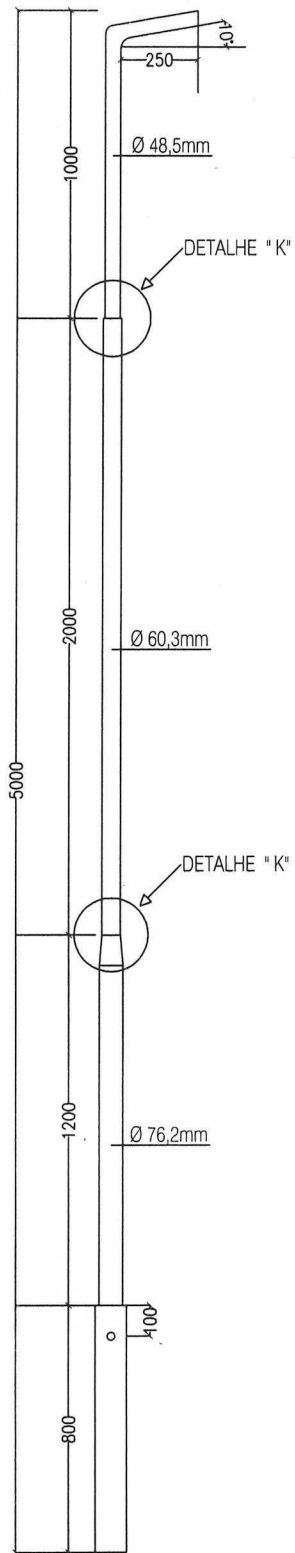
ELEVAÇÃO
